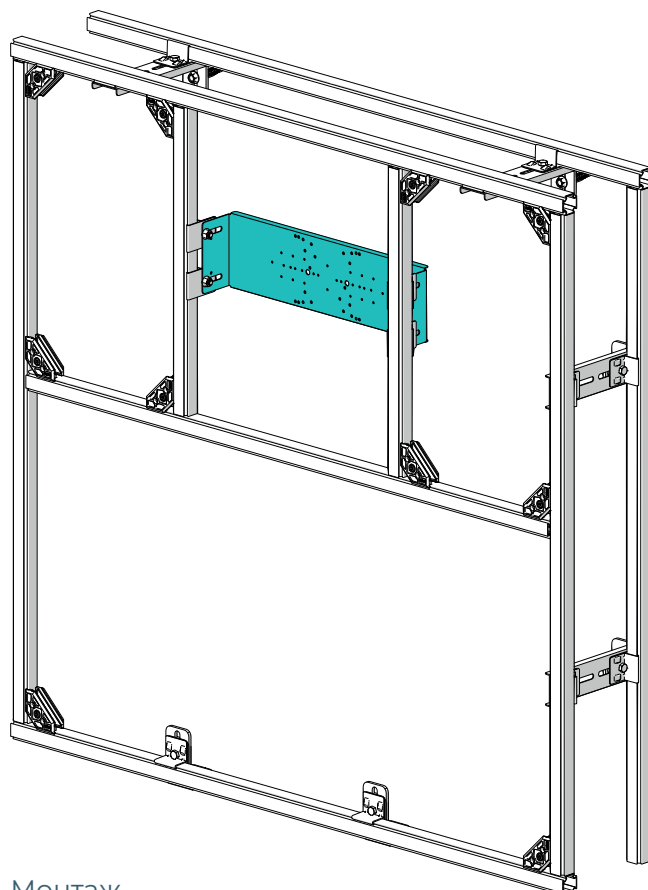
Монтаж в профиль RIVO Fix
