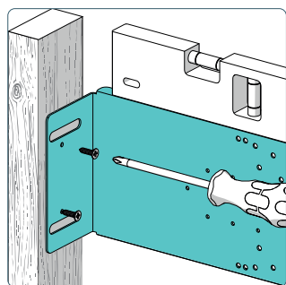
Монтаж в деревянный каркас
