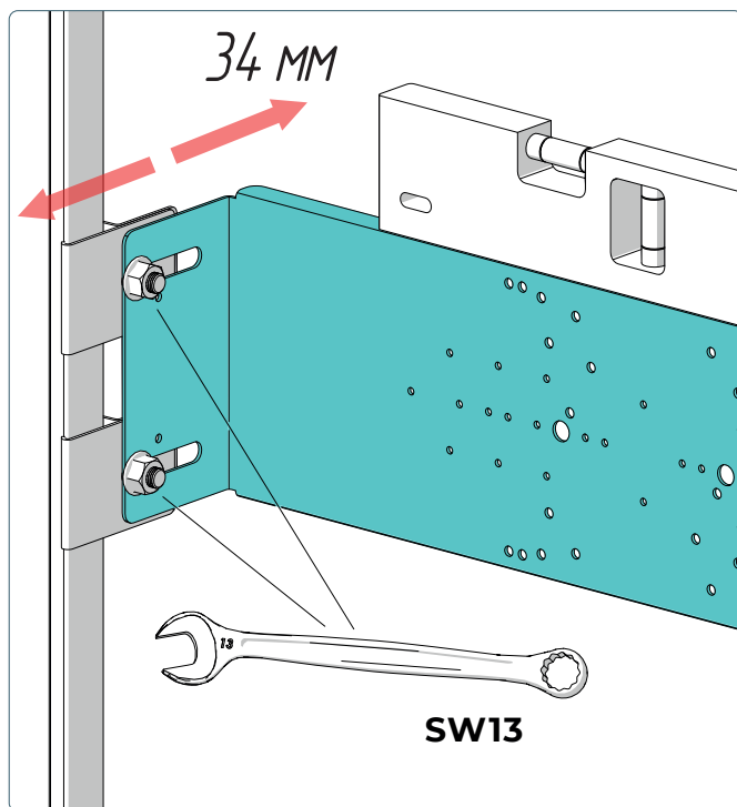
Монтаж в профиль RIVO Fix
