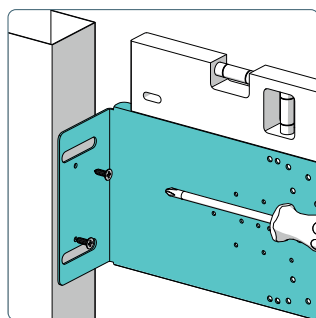
Монтаж в профиль для гипсокартона
